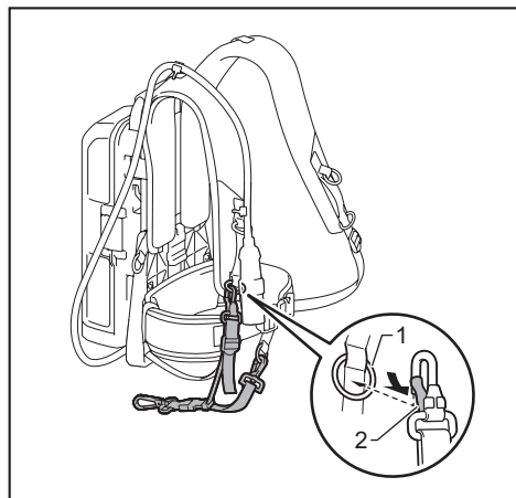
► 1. Ring 2. Hook
